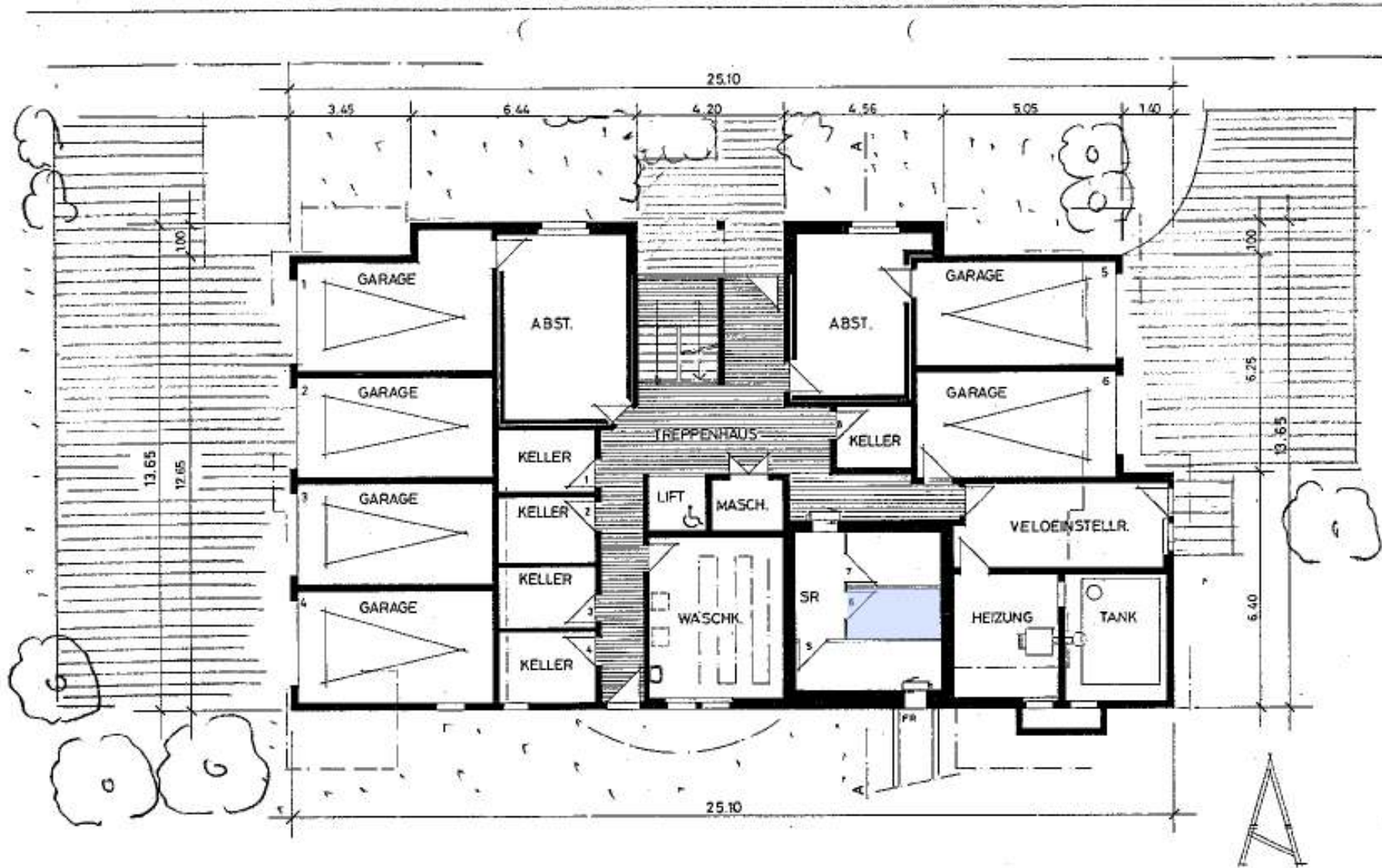
GRUNDRISS ERDGESCHOSS 1:100 16.02.95 95/11
