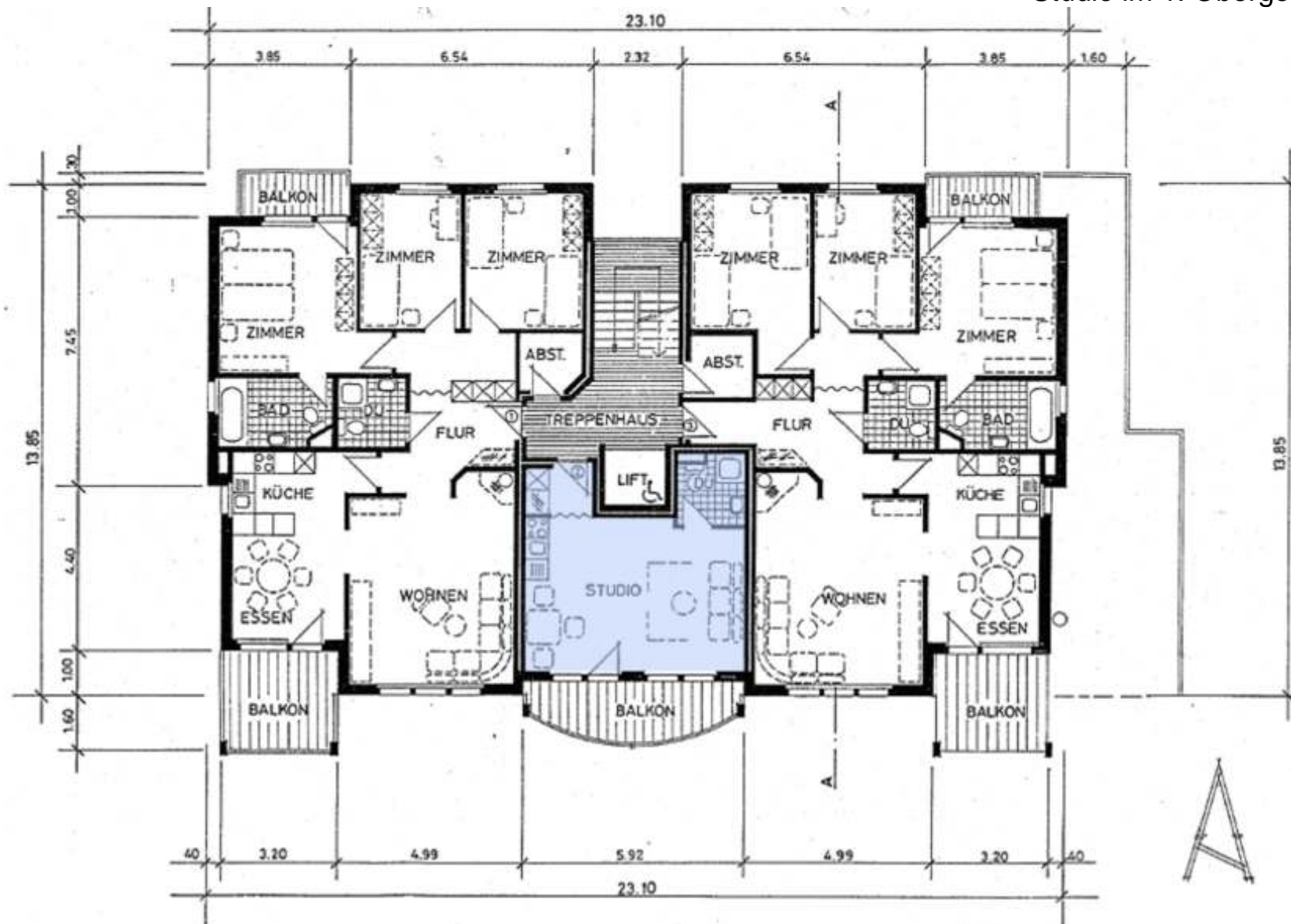
GRUNDRISS 1. OBERGESCHOSS 1:100 16.02.95 95/11
